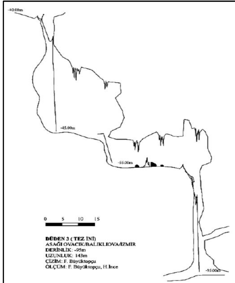
Şekil 1. 10: Tezini Mağarası Krokisi
