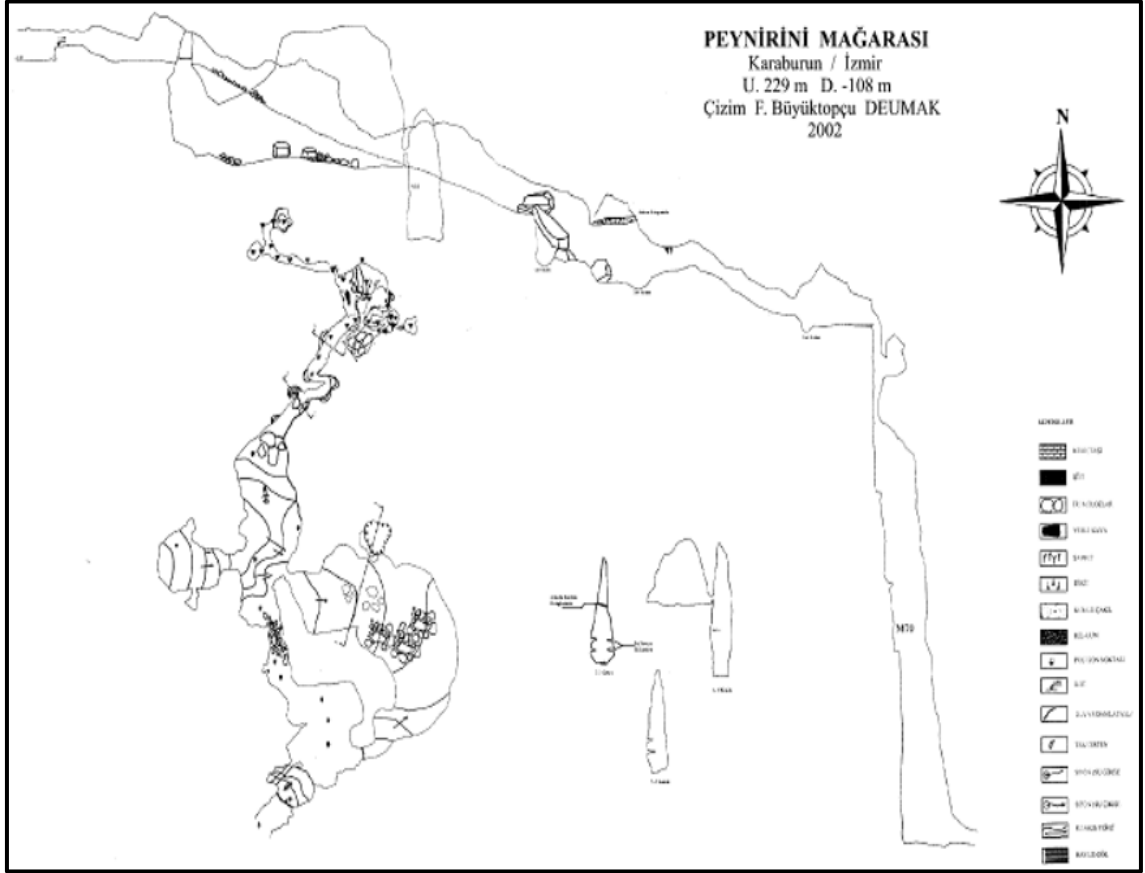
Şekil 1. 9: Peynirini Mağarası Krokisi
