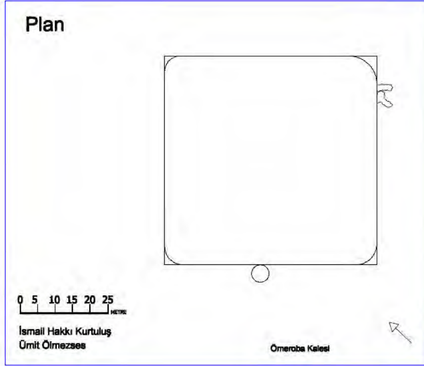
Çiz. 24. Ömeroba köyündeki kalenin planı (İ.H.Kurtuluş, Ü. Ölmezses, 2019).
