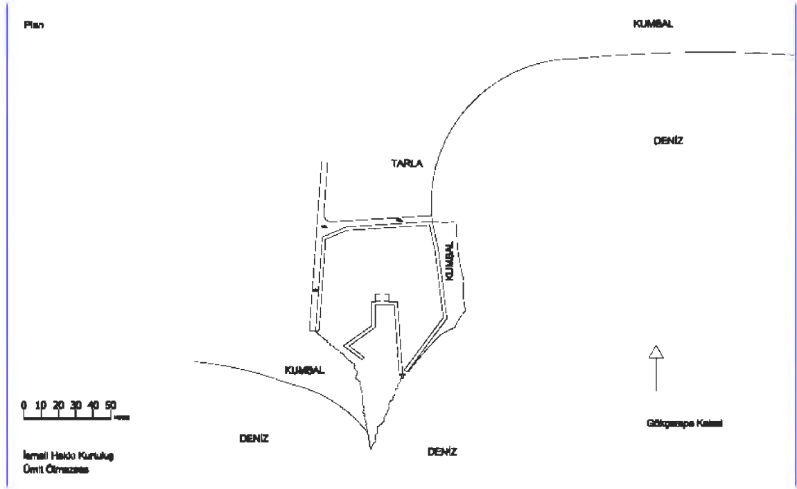
Çiz. 39. Gökçetepe Kalesinin Planı (İ.H. Kurtuluş, Ü. Ölmezses, 2019)
