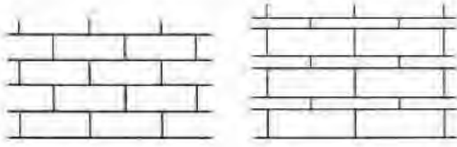
Çiz. 16. İso-domik ve pseudo isodomic duvar.
