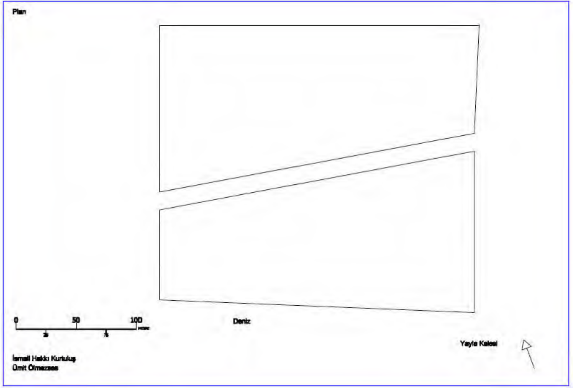
Çiz. 42. Yaylaköy Kalesinin Planı (İ.H. Kurtuluş, Ü. Ölmezses, 2019)
