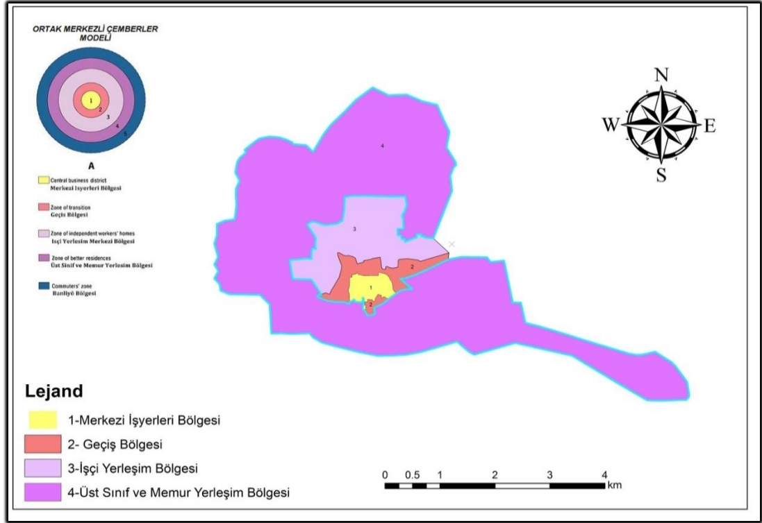
Şekil 3.6: Ortak Merkezli Çemberler Modelinin Kilis Şehrine Uygunluğu.
