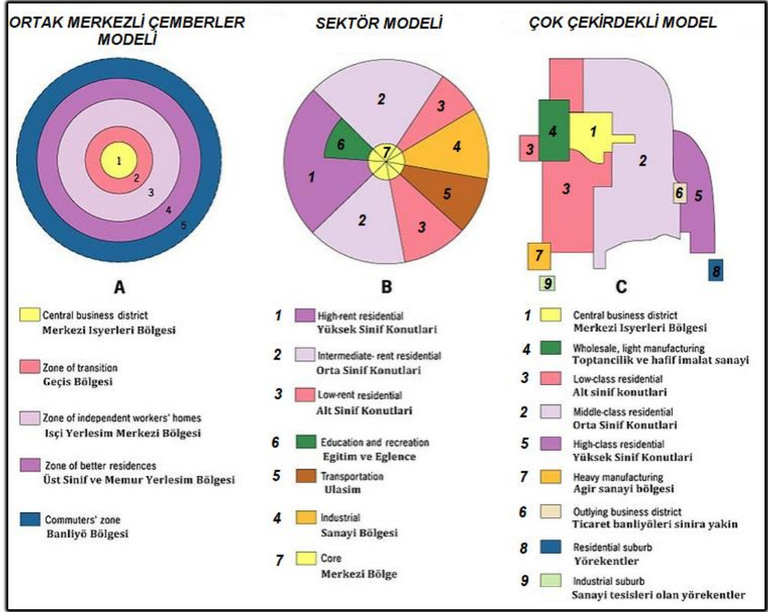
Şekil 3.5: Şehir İçi arazi Kullanım Modelleri.
