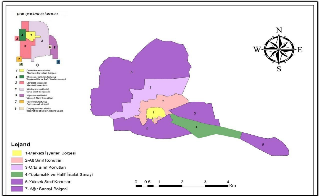
Şekil 3.8: Çok Çekirdekli Modelinin Kilis Şehrine Uygunluğu.
