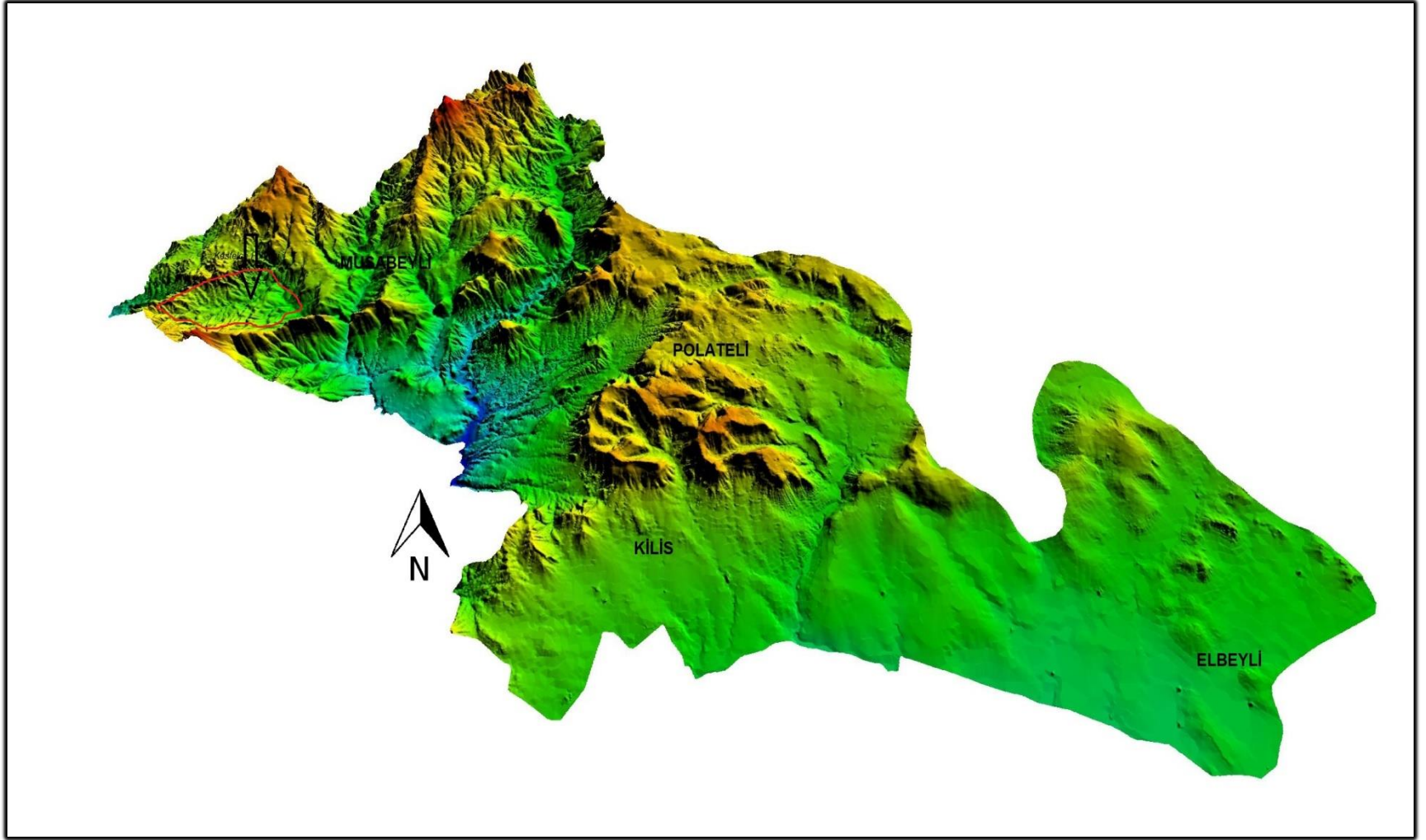
Şekil 1.1: Kilis İlinin Blokdiagramı.
