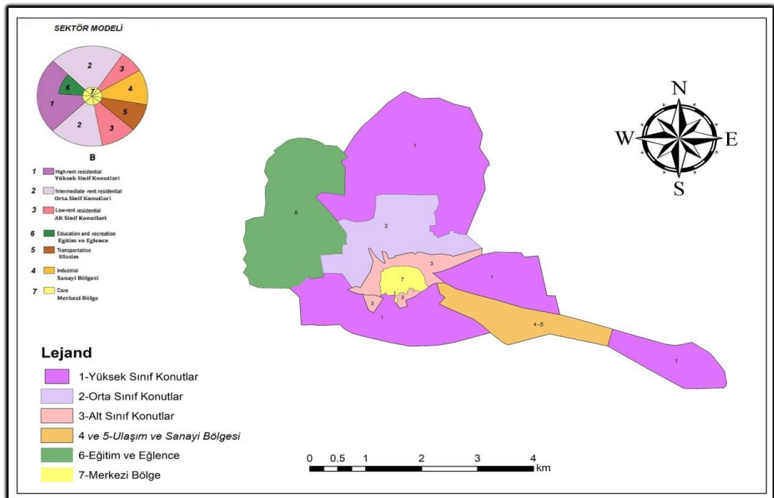
Şekil 3.7: Sektör Modelinin Kilis Şehrine Uygunluğu.
