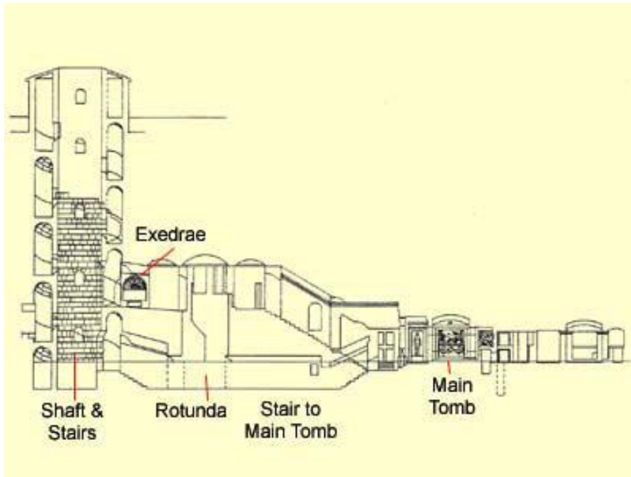
Resim 113. Kom eş-Şokafa Katakombları – Plan 598
