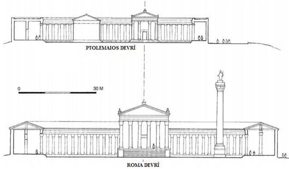
Resim 110. Aleksandreia Sarapaionu – Ptolemaios ve Roma Devri Rekonstrüksyon Enine Kesidi 596
