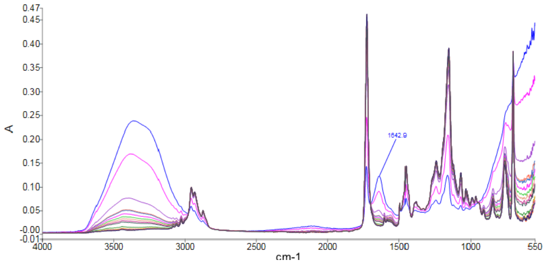
Şekil 4.29: Zamana bağlı su absorban değerinin azalması.
