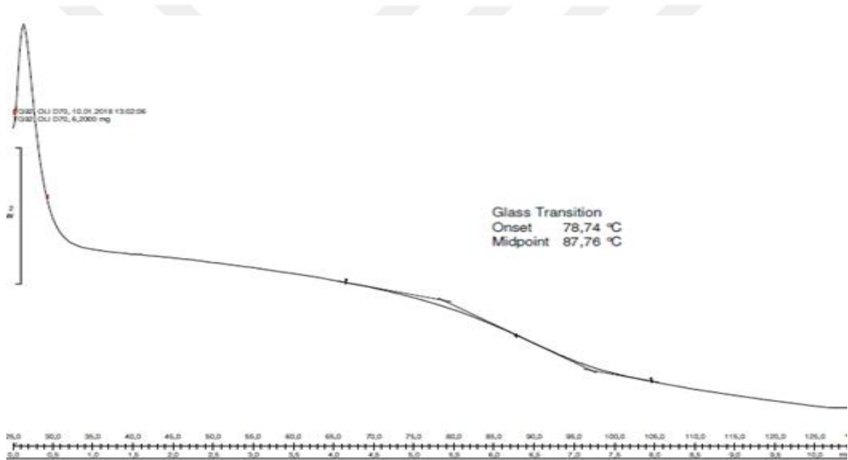
Şekil 4.1: Deneme 13 (AÇR-N)'e ait DSC grafiği.
