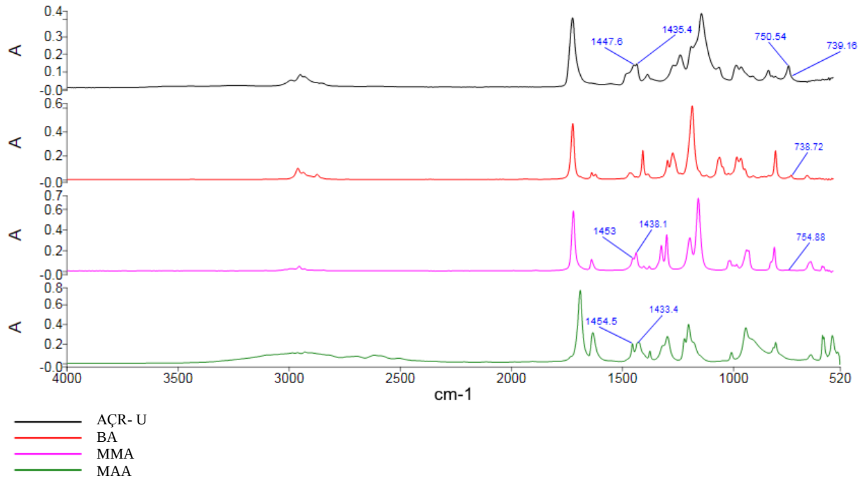
Şekil 4.11: MMA/MAA/BA bileşiminde hazırlanmış AÇR ve yapıyı oluşturan monomerlerin FTIR spektrumları.
