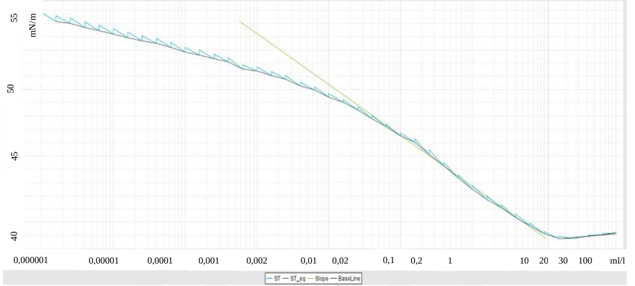
Şekil 4.14 : MMA-MAA-ST AÇR'nin konsantrasyona bağlı yüzey gerilimi grafiği.(AÇR-N konsantrasyonuna bağlı olarak yüzey geriliminin değişimi).
