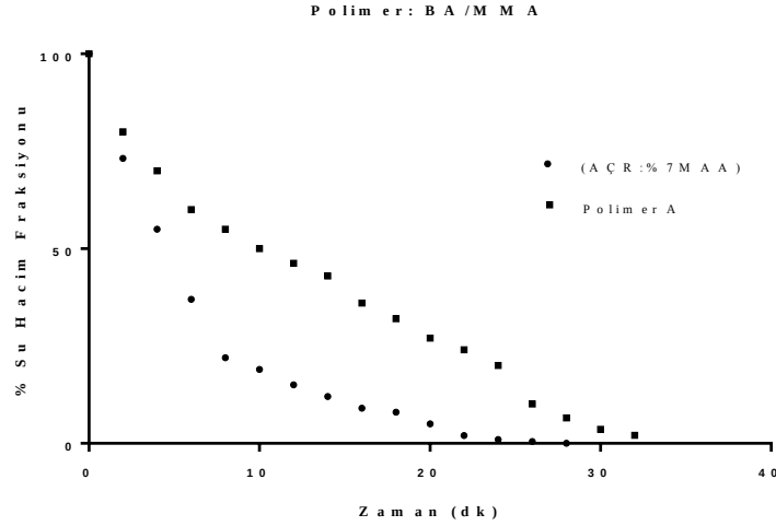
Şekil 4.30: Farklı sürfaktanlar (AÇR – Anyonik) kullanılarak sentezlenen polimerlerde suyun zamana bağlı hacim fraksiyonu azalması.
