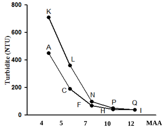
Şekil 4.6: MAA oranı ile iki gruptaki (ST ve EA) ürünlerin bulanıklıklarının değişimi.
