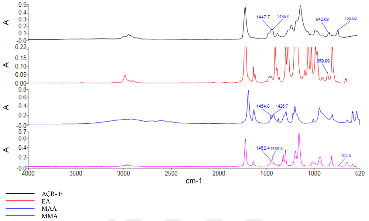
Şekil 4.8: MMA/MAA/EA bileşiminde hazırlanmış AÇR ve yapıyı oluşturan monomerlerin FTIR spektrumları.
