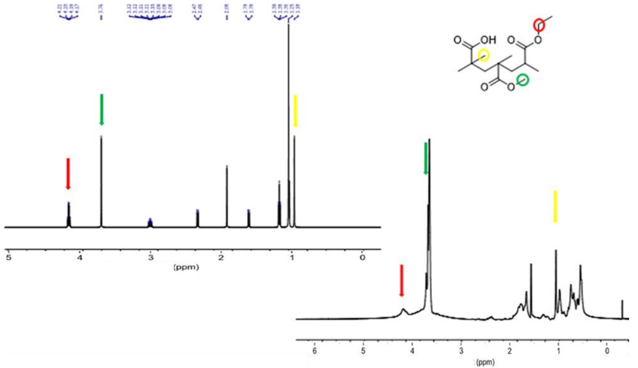
Şekil 4.12: MMA-MAA-EA monomer kompozisyonuna sahip AÇR'nin NMR spektrumları.
