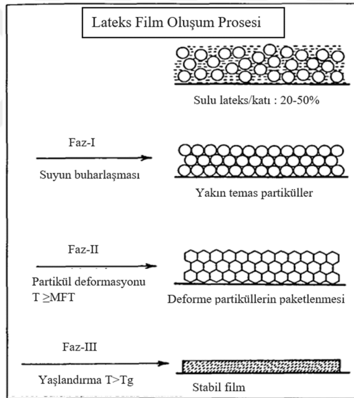
Şekil 2.3: Lateks film oluşum proses şeması.
