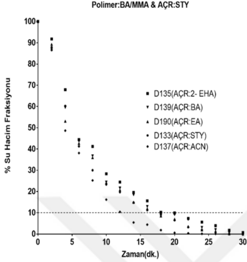
Şekil 4.33: Farklı Tg değerlerine sahip polimerlerdeki suyun zamana bağlı hacim fraksiyonu
