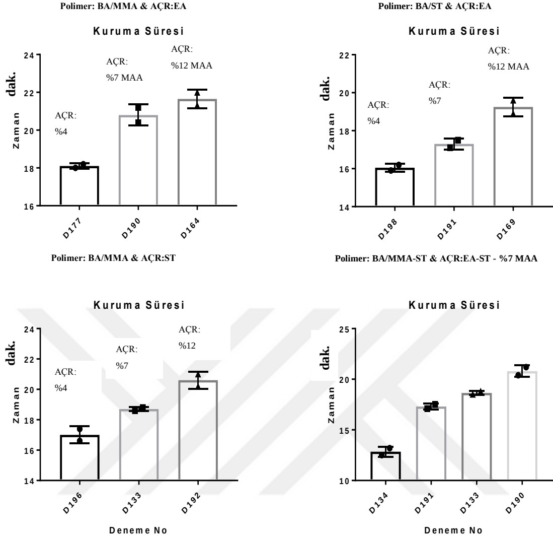
Şekil 4.32: Farklı hidrofilitedeki polimerlerde film kazıma yöntemi ile kuruma zamanı kayıt cihazı değerleri
