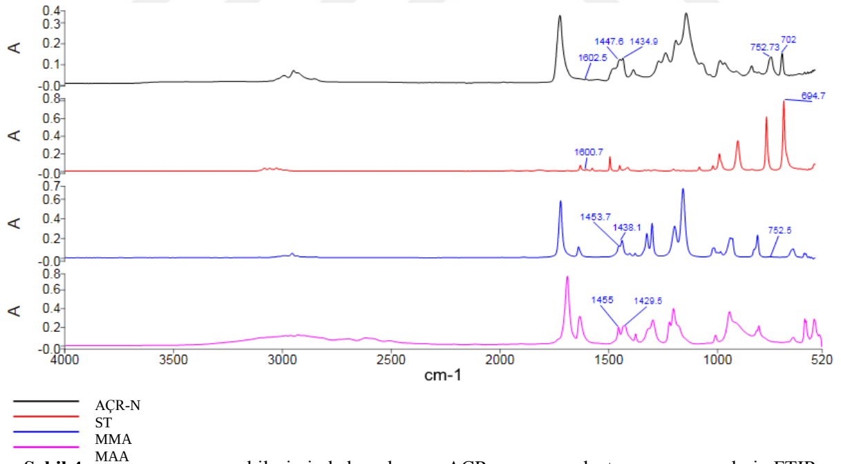
Şekil 4.7. MMA/MAA/EA bileşiminde hazırlanmış AÇR ve yapıyı oluşturan monomerlerin FTIR spektrumları.
