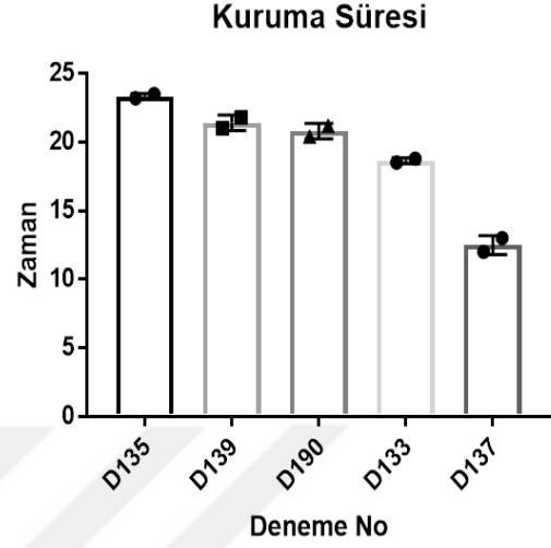
Şekil 4.34: Farklı Tg değerlerine sahip polimerlerdeki film kazıma yöntemi ile kuruma zamanları
