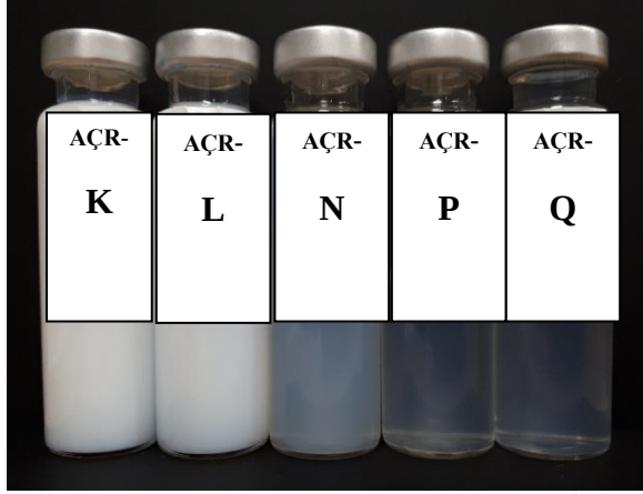
Şekil 4.2: Farklı MAA oranına sahip ST/MMA bazlı AÇR'nin alkalide çözünme sonrası görüntüleri.
