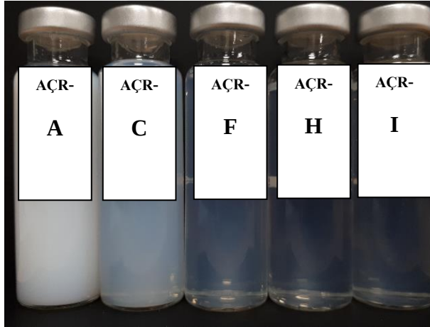
Şekil 4.3: Farklı MAA oranına sahip EA/MMA bazlı AÇR'nin alkalide çözünme sonrası görüntüleri.
