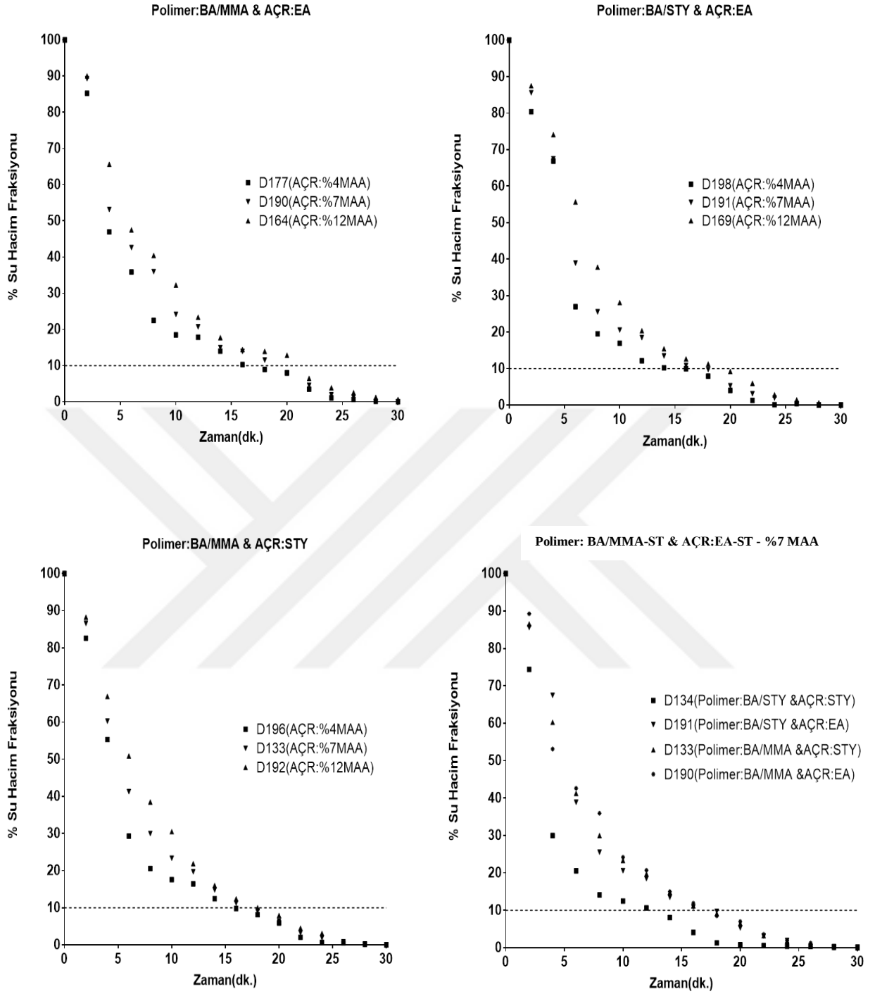
Şekil 4.31: Farklı hidrofilitedeki polimerlerde suyun zamana bağlı hacim fraksiyonu azalması
