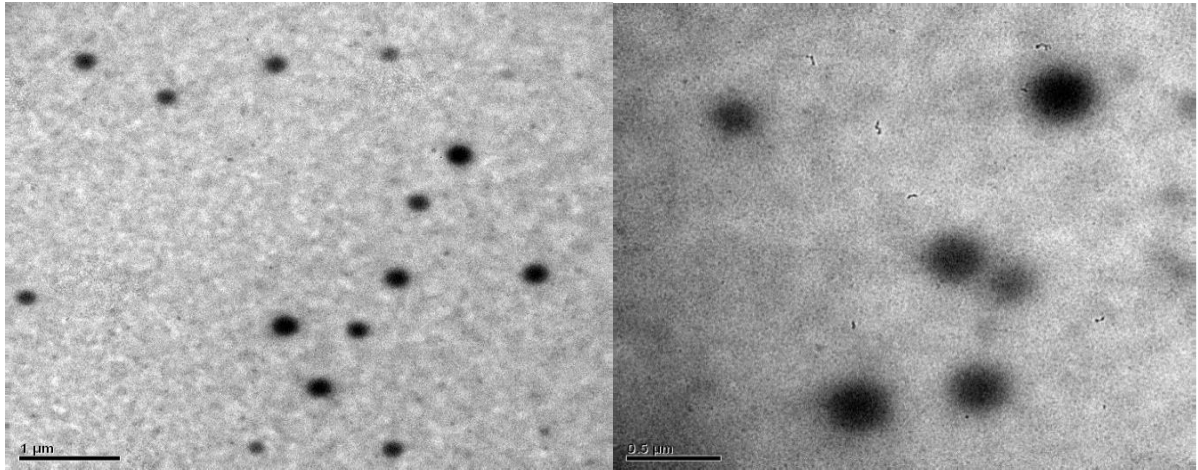
Şekil 4.24: Deneme 191, 1 µm ve 0,5 µm TEM görüntüleri.
