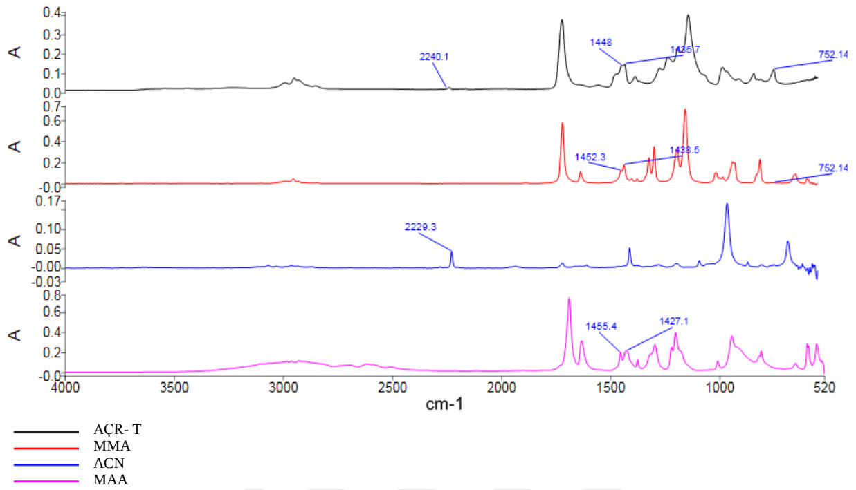
Şekil 4.10: MMA/MAA/ACN bileşiminde hazırlanmış AÇR ve yapıyı oluşturan monomerlerin FTIR spektrumları.
