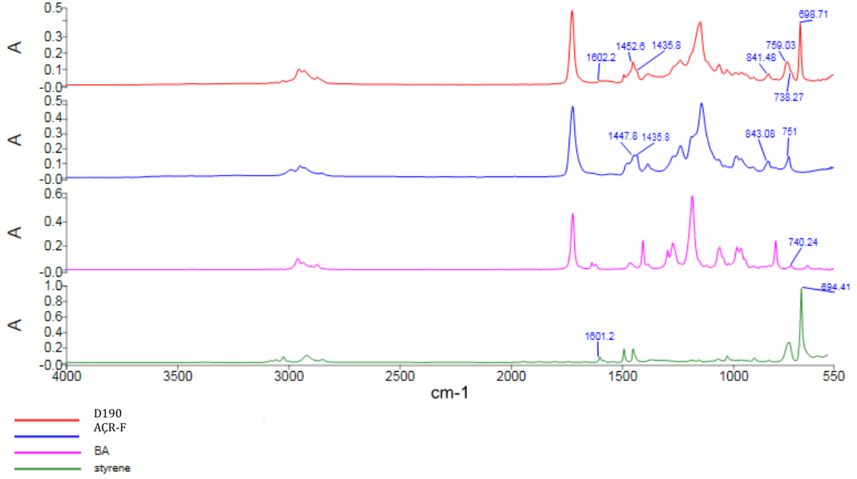
Şekil 4.26: BA/ST bileşiminde hazırlanmış polimer ve yapıyı oluşturan monomerlerin FTIR spektrumları.
