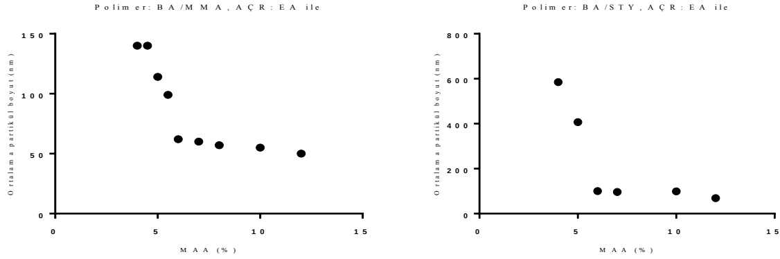
Şekil 4.19: AÇR’lerdeki MAA oranının polimerin ortalama partikül büyüklüğüne etkisi.
