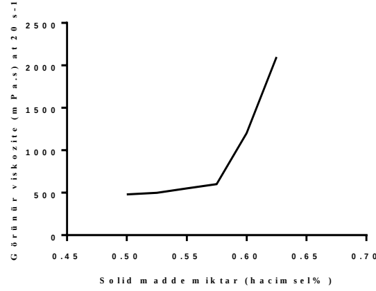
Şekil 2.1: Katı madde içeriğinin bir fonksiyonu olarak lateksin 20 s -1 'lik bir sabit kesme hızında viskozitesi (katı madde yüzde olarak gösterilmiştir).
