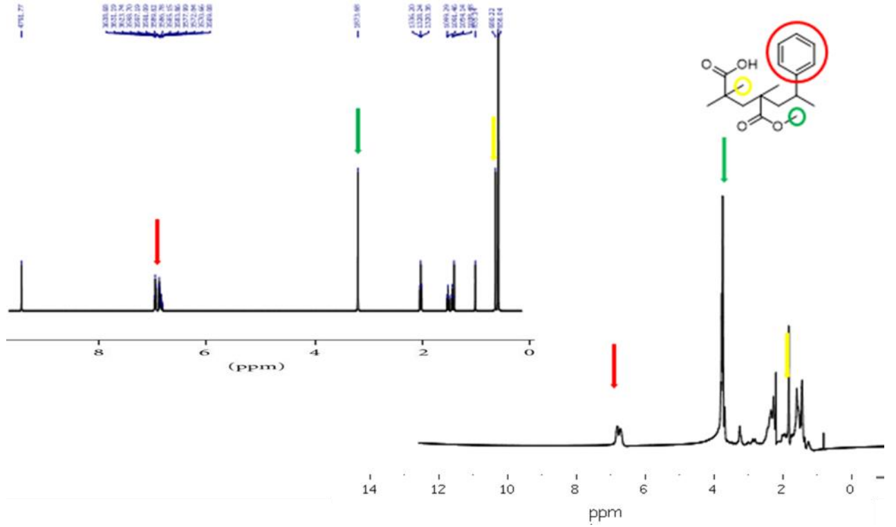
Şekil 4.13: MMA-MAA-ST monomer kompozisyonuna sahip AÇR'nin NMR grafikleri.
