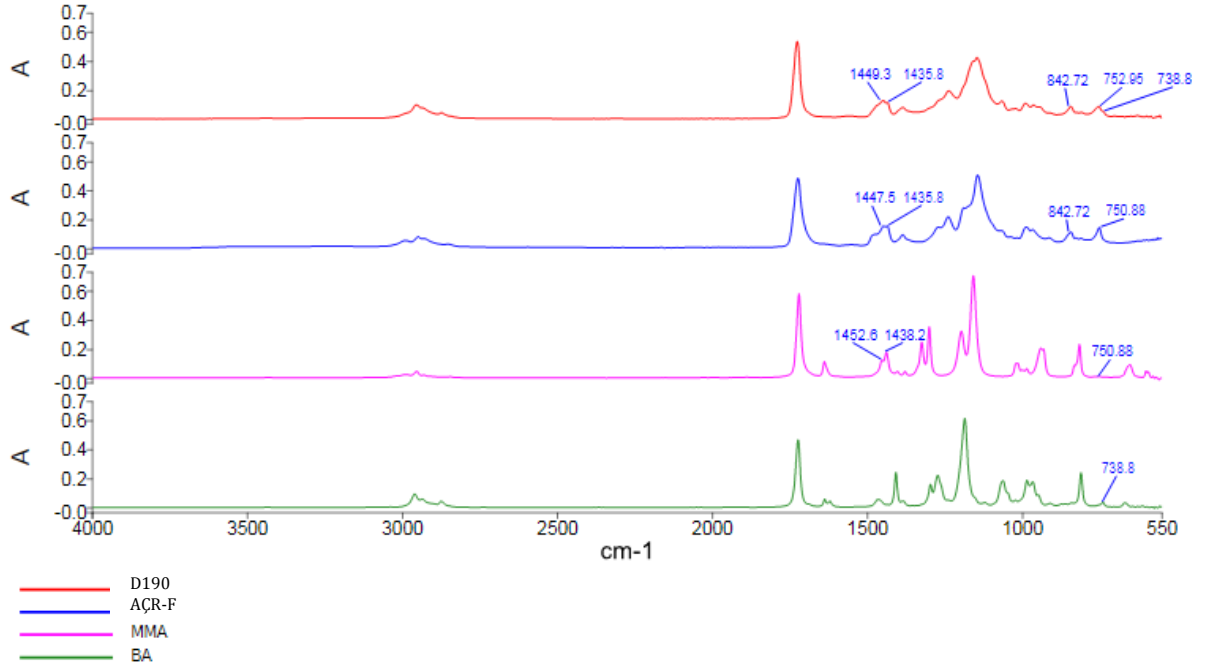
Şekil 4.25: BA/MMA bileşiminde hazırlanmış polimer ve yapıyı oluşturan monomerlerin FTIR spektrumları.
