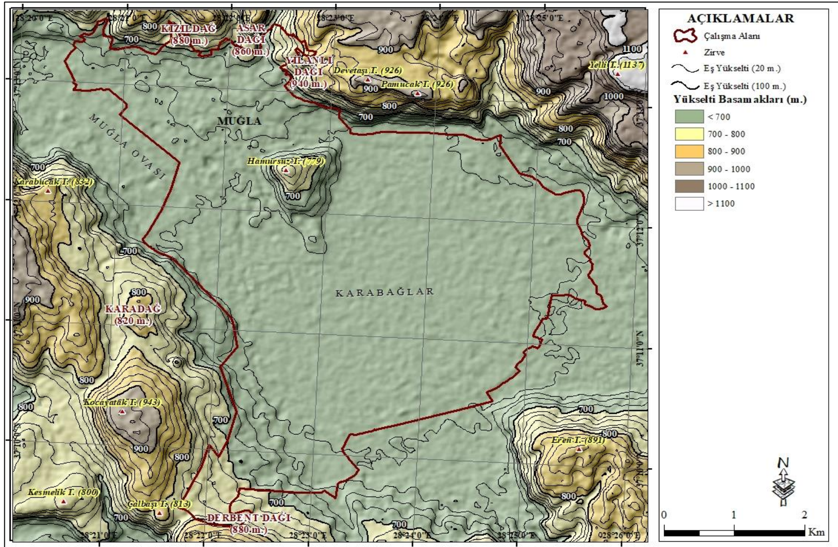
Şekil 11: Muğla Kenti ve Çevresinin Topografyası
