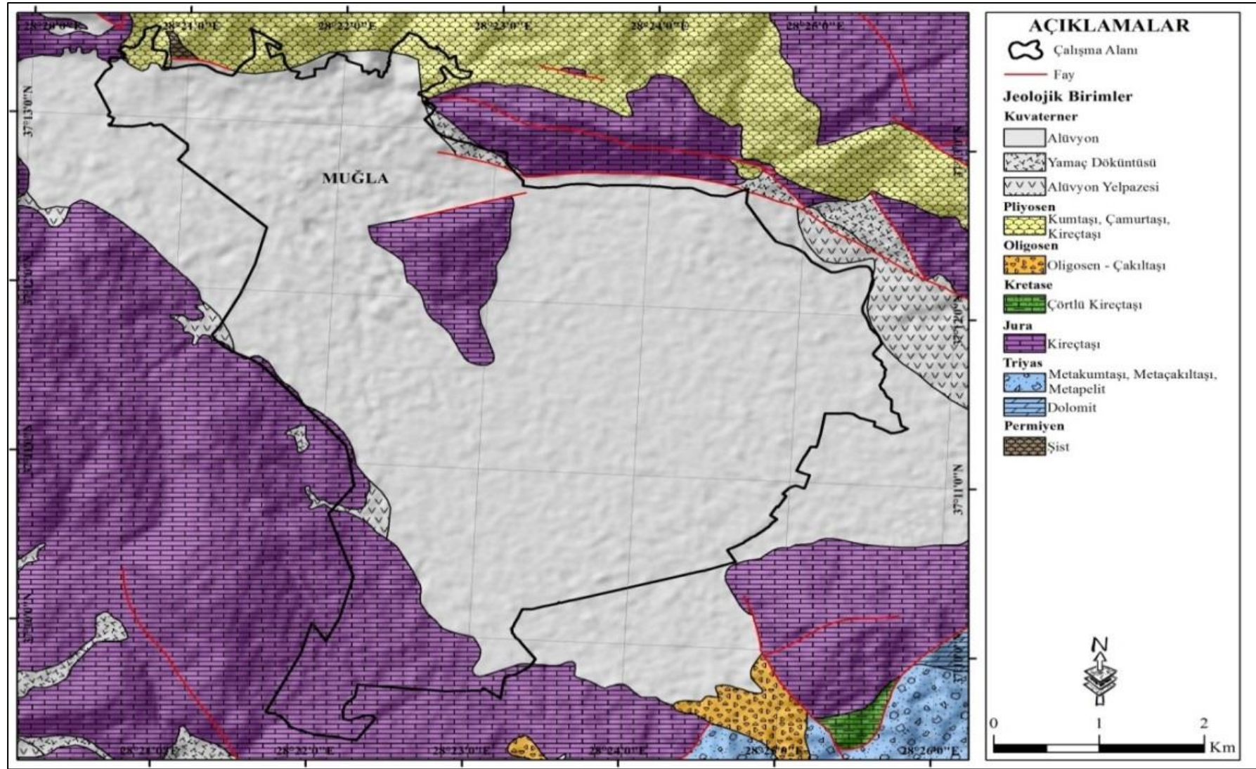
Şekil 10: Muğla Kenti ve Çevresinin Jeolojisi
