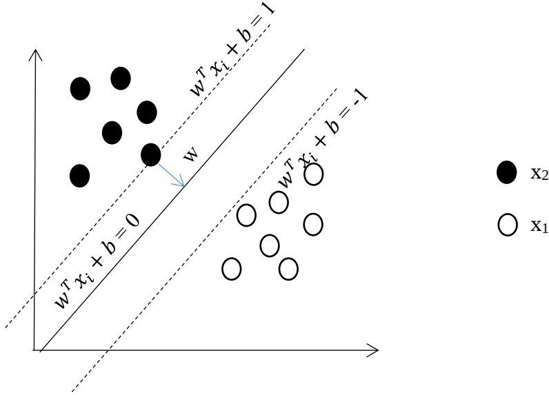
Şekil 6: Karar destek makineleri algoritması
