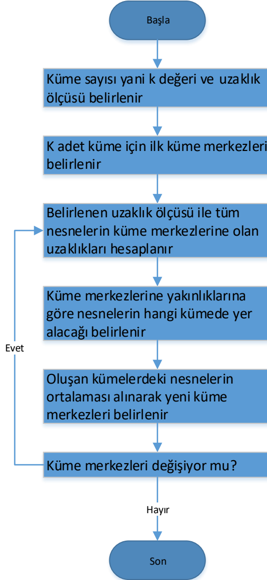
Şekil 7: K-ortalamalar algoritması
