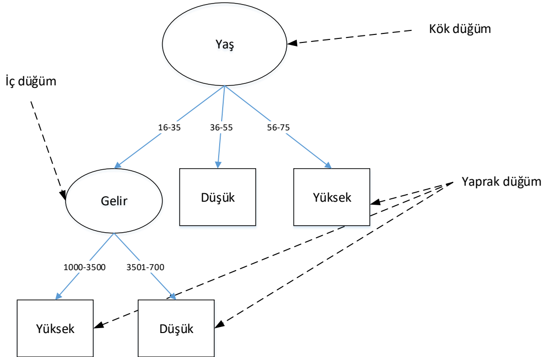
Şekil 3: Karar ağacı algoritması
