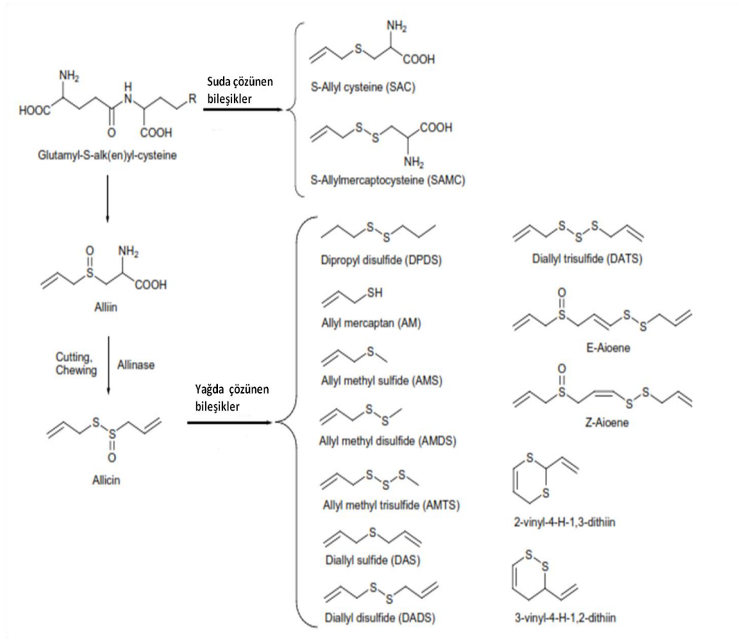
Şekil 2.10: Sarımsakta yaygın olarak incelenen organosülfür bileşiklerinin kimyasal yapıları [88].
