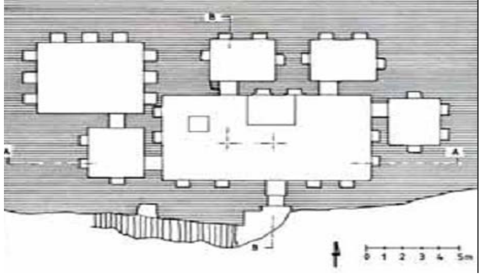
Plan 1: I. Arğişti oda mezarı planı
