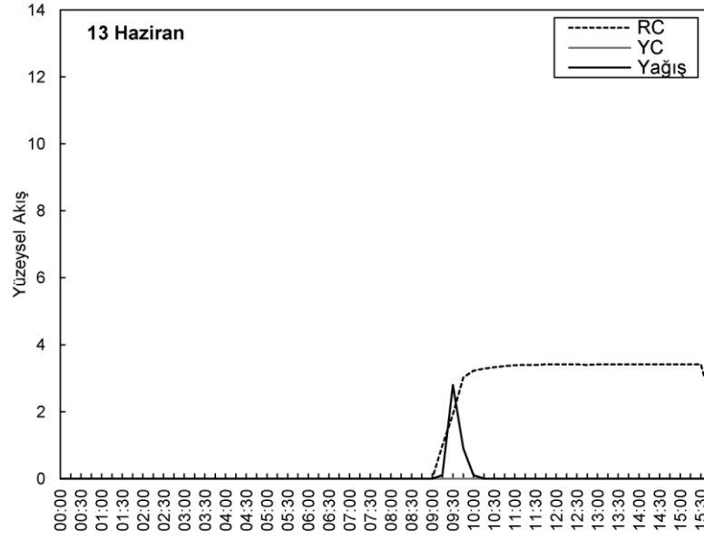
Şekil 4.52: 13 Haziran 2011 tarihindeki yağış miktarı ile yüzeysel akışın karşılaştırılması
