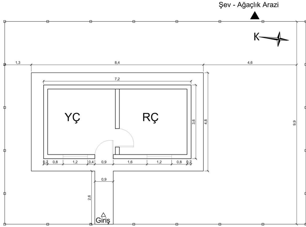
Şekil 3.3: Araştırma alanı planı ve ölçüleri
