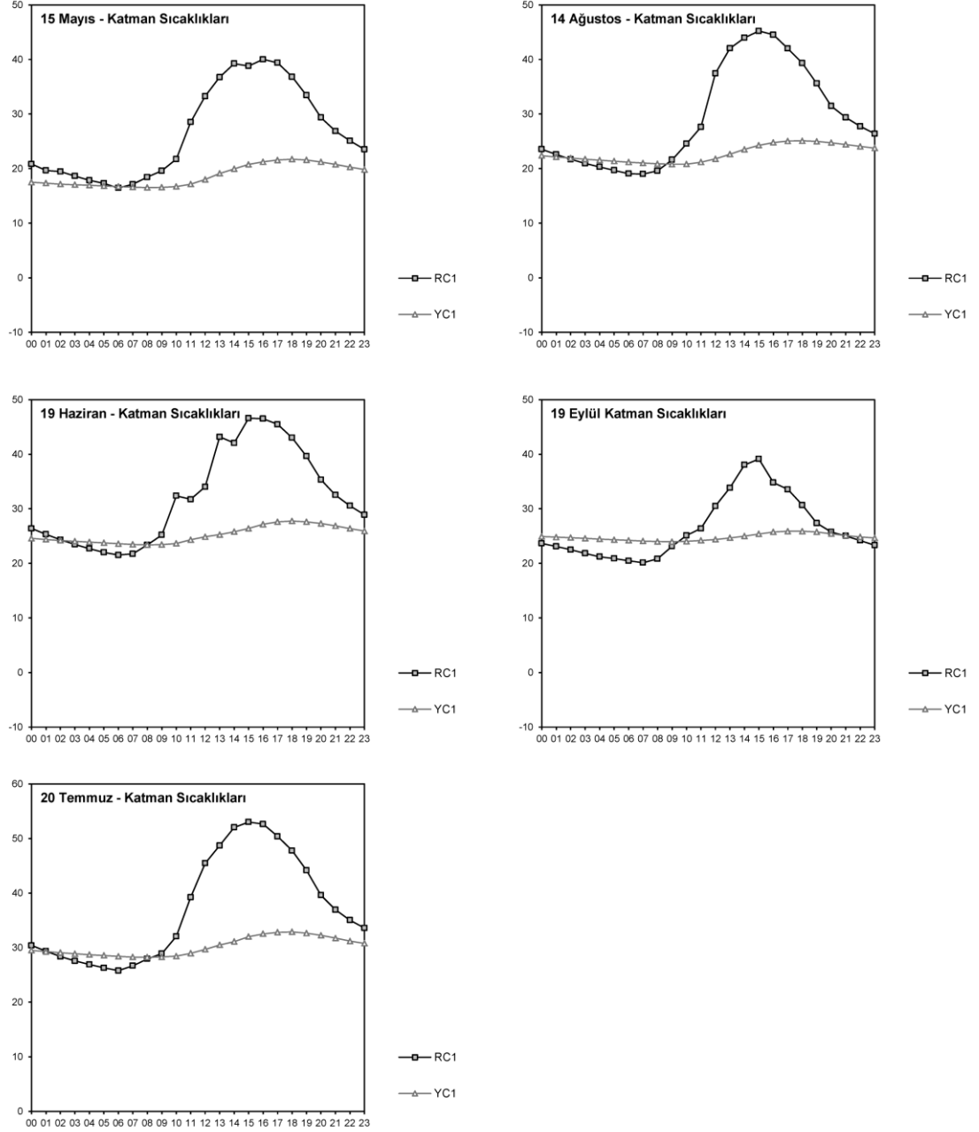
Şekil 4.26: Ölçüm dönemi içerisinde rastgele seçilen günlerde oluşan çatı levhası sıcaklıkları
