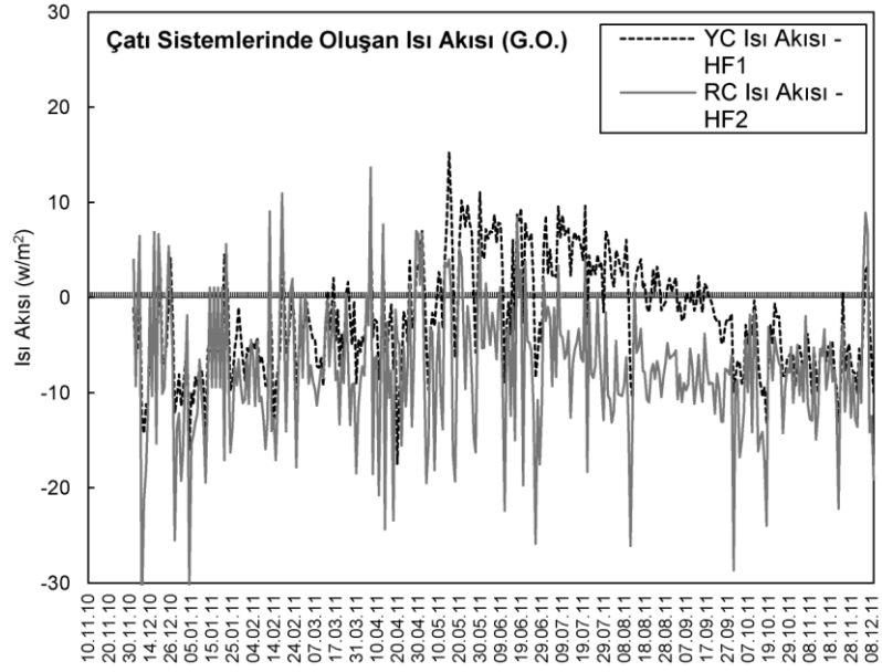
Şekil 4.27: Her iki çatı sisteminde oluşan günlük ortalama ısı akısı miktarı
