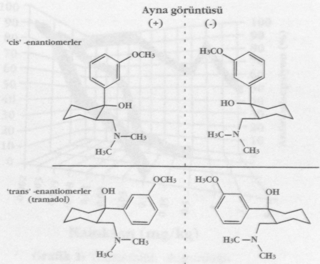
Şekil 2: Tramadolün enantiomerleri.
