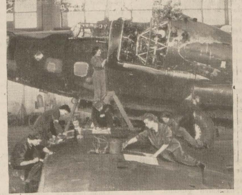
Bu resim müttefiklerin hava ordusunun bir atelyesini göstermektedir. Kız işçilerin bazıları, tayyare motorünü temizlemekte, bazıları da bir "Vellington" tayyaresinin kanadını tamir etmektedir.
