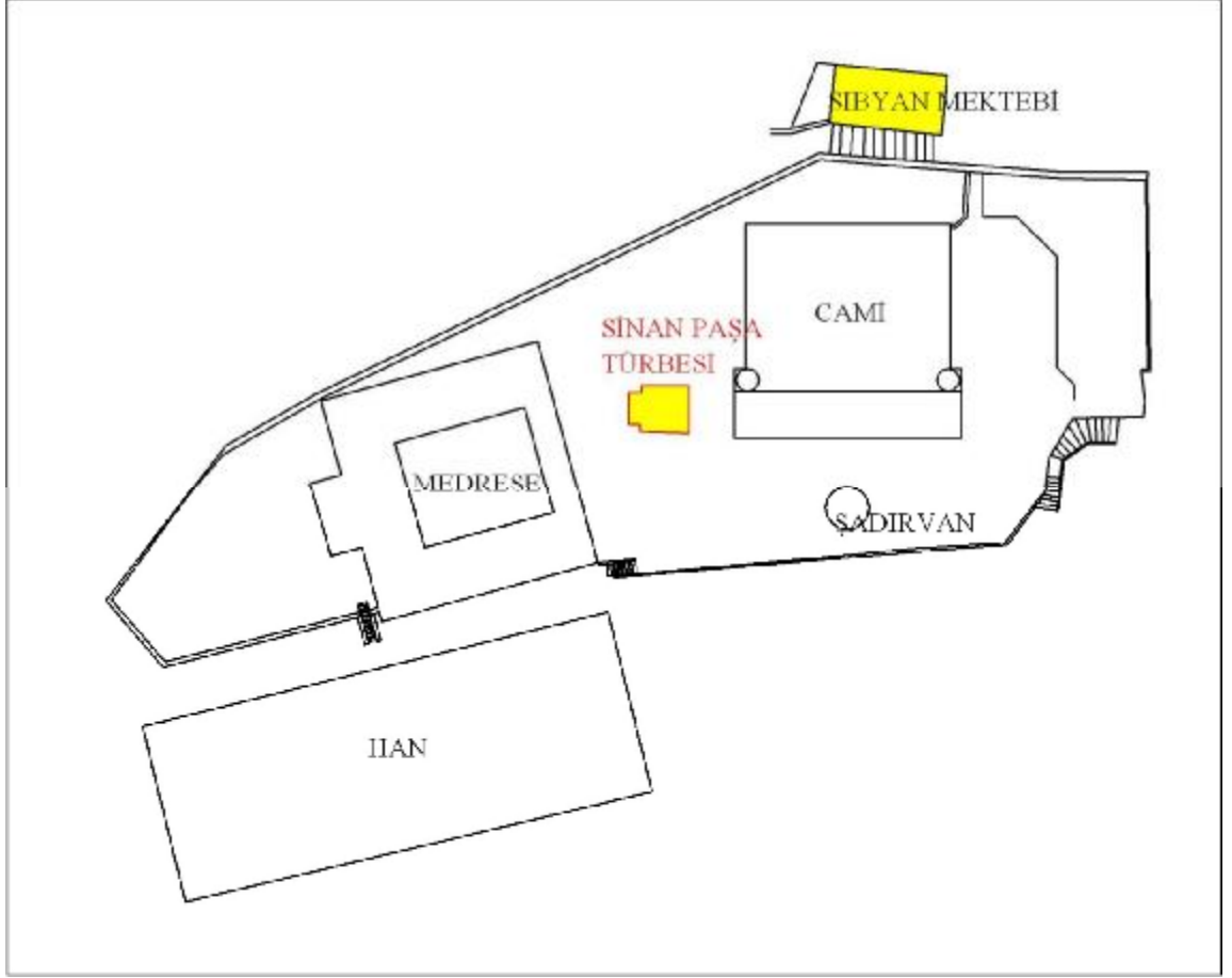
Çizim 2 Üsküdar Mihrimah Sultan Külliyesi Plan Oluşum Şeması 961h (1553m) yılı
