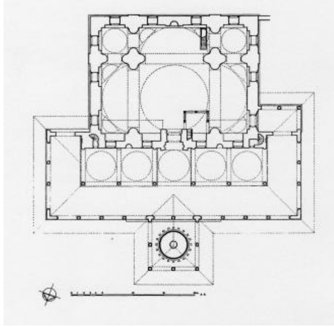
Çizim 9 Üsküdar Mihrimah Sultan Camii planı
