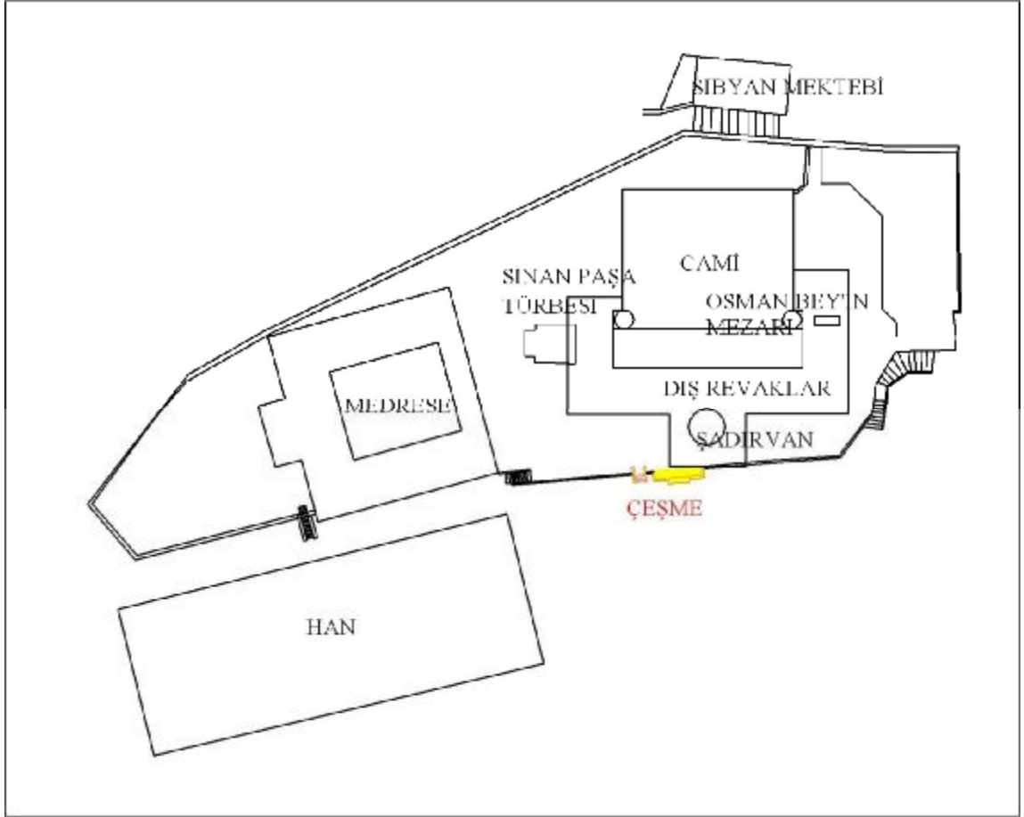
Çizim 4 Üsküdar Mihrimah Sultan Külliyesi Plan Oluşum Şeması 1092h (1681m) yılı
