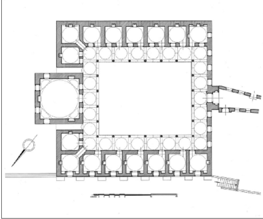
Çizim 10 Üsküdar Mihrimah Sultan Merdesesi planı
