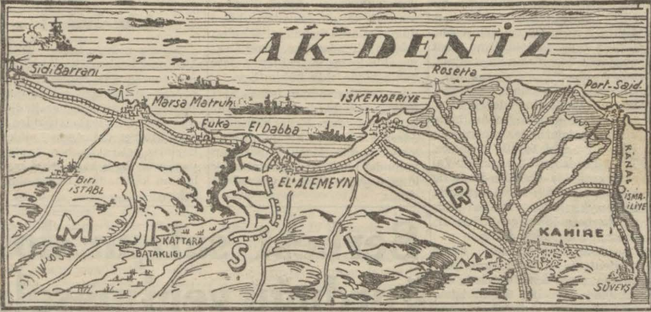
Mısırda sekizinci ordunun giriştiği büyük taarruzun istikametini gösteren harita
