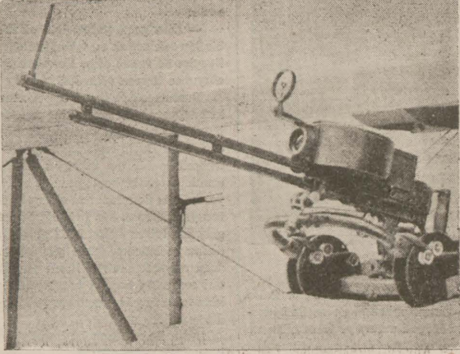
Fotoğraflı makineli tüfek bir tayyarenin üzerinde
