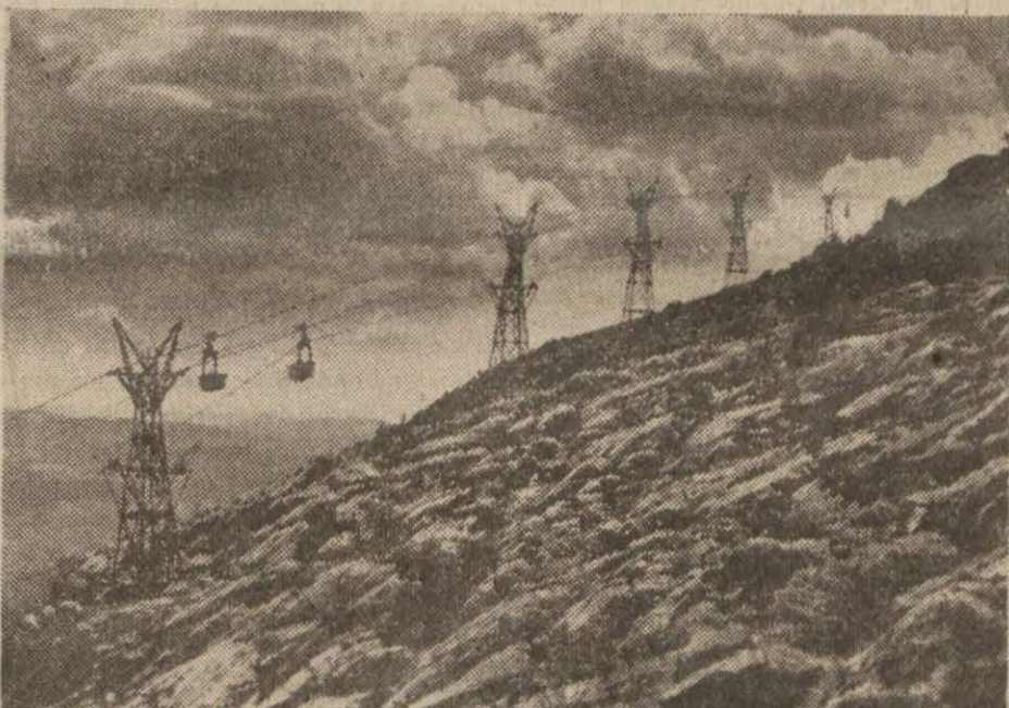
Guleman'da havai hatla maden cevheri naklediliyor
