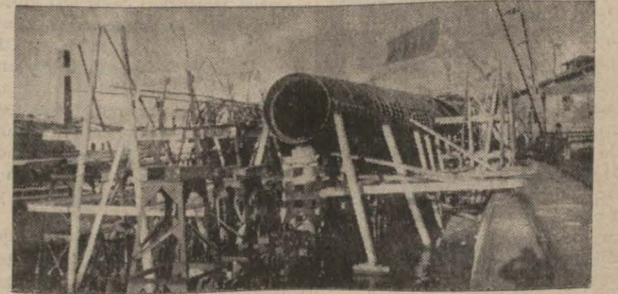
İstanbul'da iki denizaltı gemimizin inşa edilmekte olduğunu telefon haberi olarak bildirmiştik. Yukarıdaki resimde denizaltıların inşaatı görülmektedir
