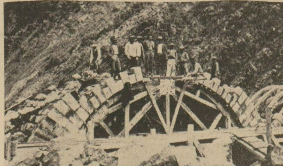
Sivas — Erzurum demiryolu üzerinde bir köprü inşaatı
