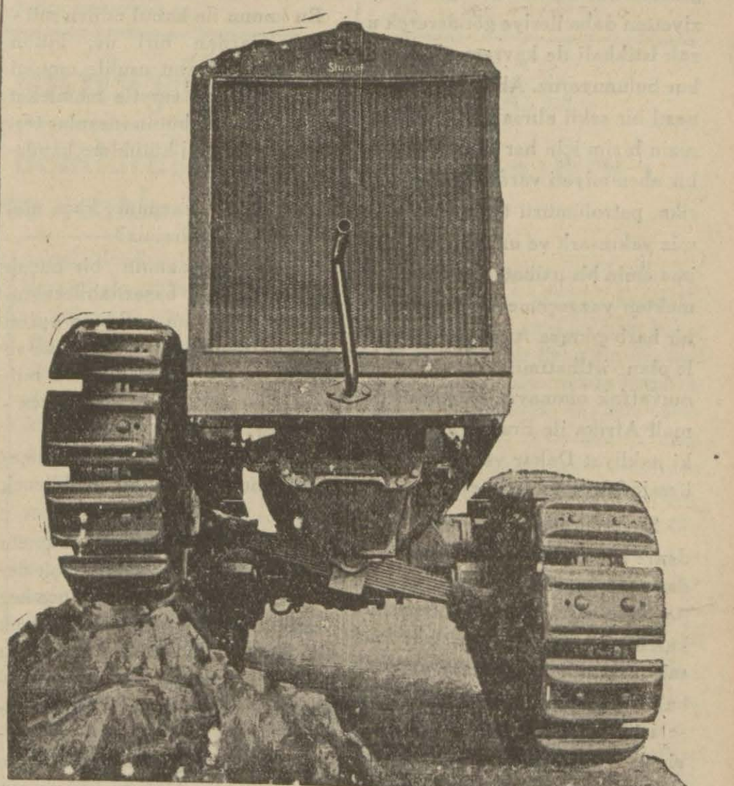
Almanların yeni imal ettikleri yük sek kudretli ordu traktörlerinden "Rübezahl,, ismini verdikleri traktörün ön taraftan görünüşü. Bu traktörün müteharrik dingilleri sayesinde en âri zali yerlerden bile kolaylıkla geçmekte olduğu bu resimde görülmektedir.
