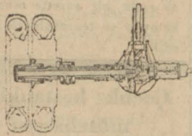
Yalnız Şevrolede bulunan masuralı tepeden motorlarla SERBEST ARKA AKSLAR
