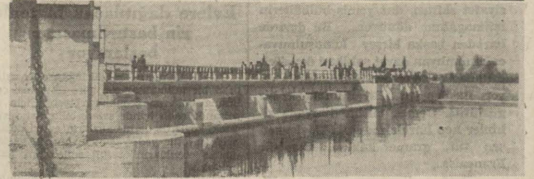
Yukarıda Nafia Vekili Ali Fuad Cebesoy Küçük Menderes tesisatını açıyor; aşağıda Küçük Menderes regülâtörü
