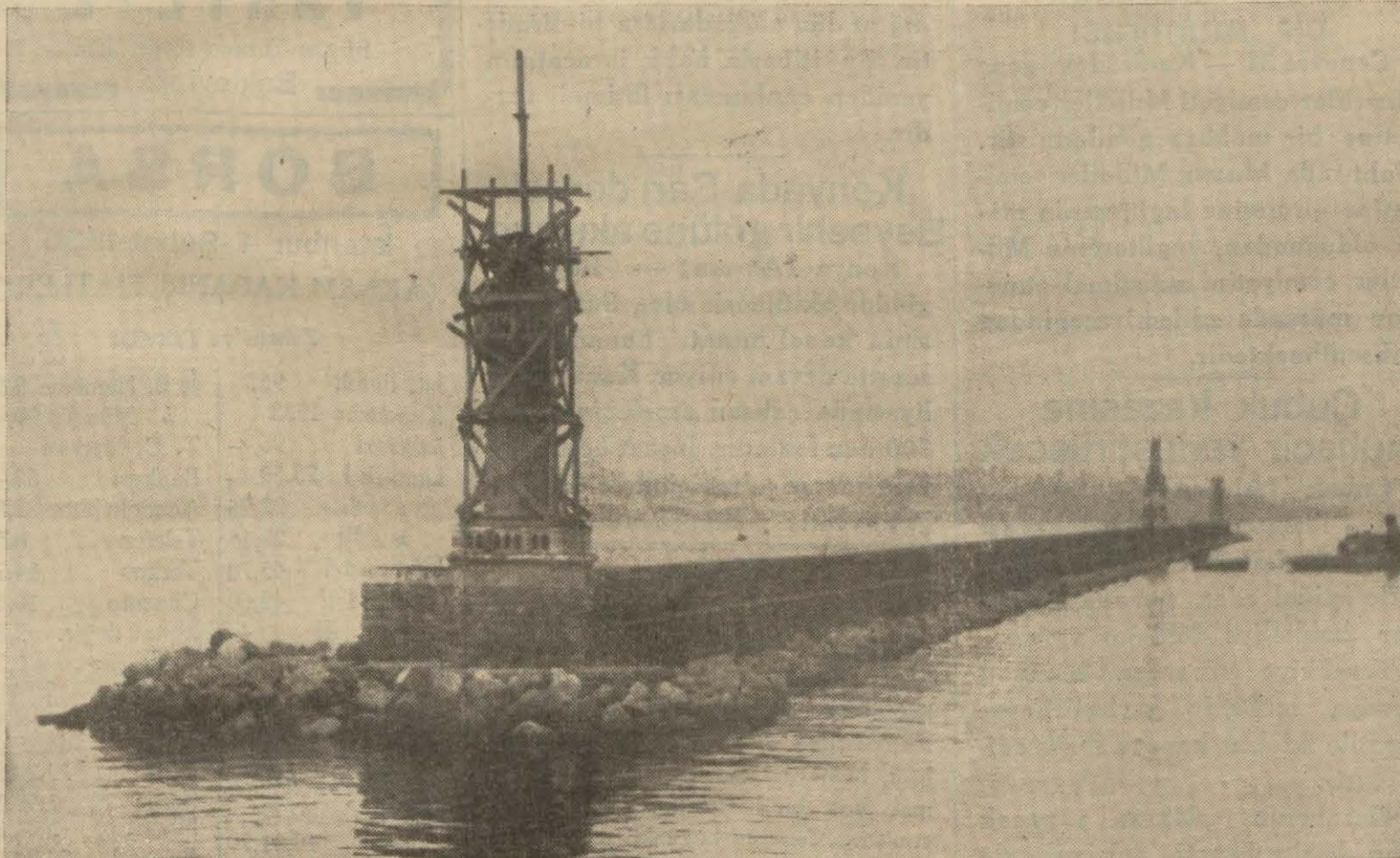
Tahlisiye idaresi sisli havalarda vapurların karaya oturmalarının önüne geçmek için Haydarpaşa dalgakıranına bir sis düdüğü koymağa karar vermiştir. Kışımız, Haydarpaşa dalgakıranı fenerinde yapılmakta olan tamirati gösteriyor.
