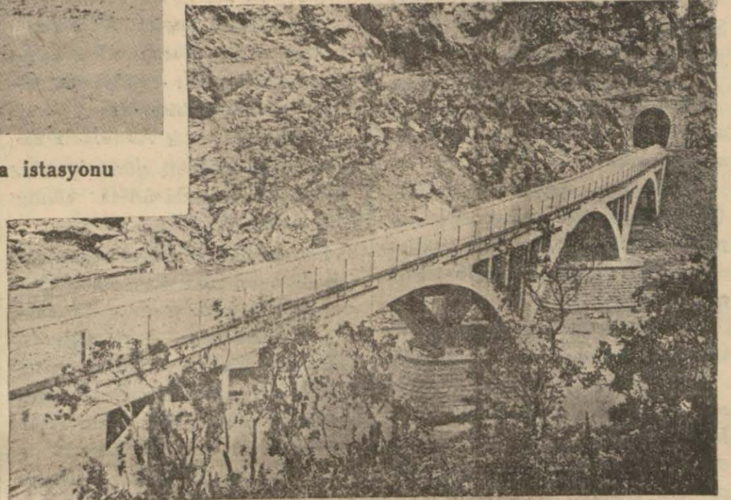
Geçen hafta açılı İrmak - Filyos hattı üzerinde 74 üncü kilometrede bir köprü ve tünel
