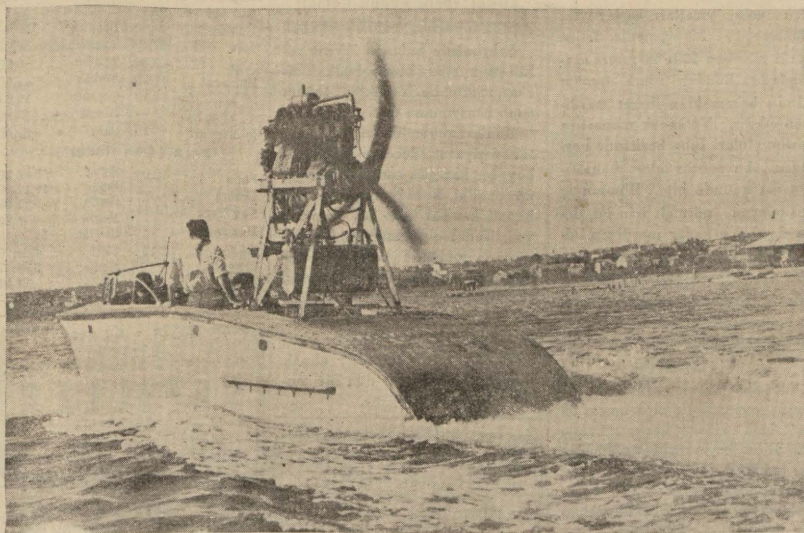
Tayyareci Vecihi bey, tayyare motörlü ile hareket eden bir motörbot yapmıştır. Bunun motörlü meydana. Yeni motörbot saatte 40 mil süratle hareket edebiliyor.
